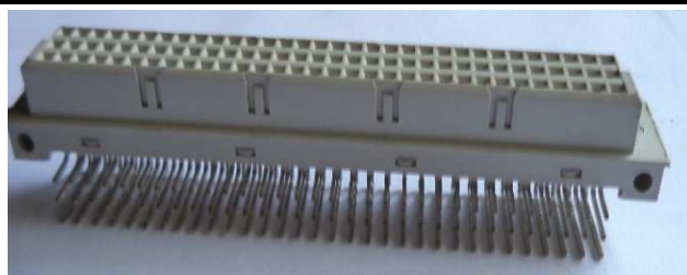
DIN 96 pinos Fêmea 90° Foto 5
